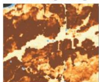
Hittestress
